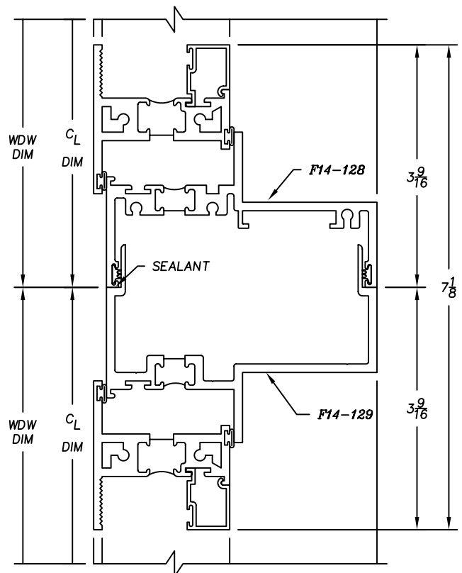
1450H SERIES - HORIZONTAL STACK F14-128 / F14-129
