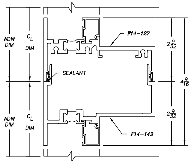
1450H SERIES - HORIZONTAL STACK F14-127 / F14-149
