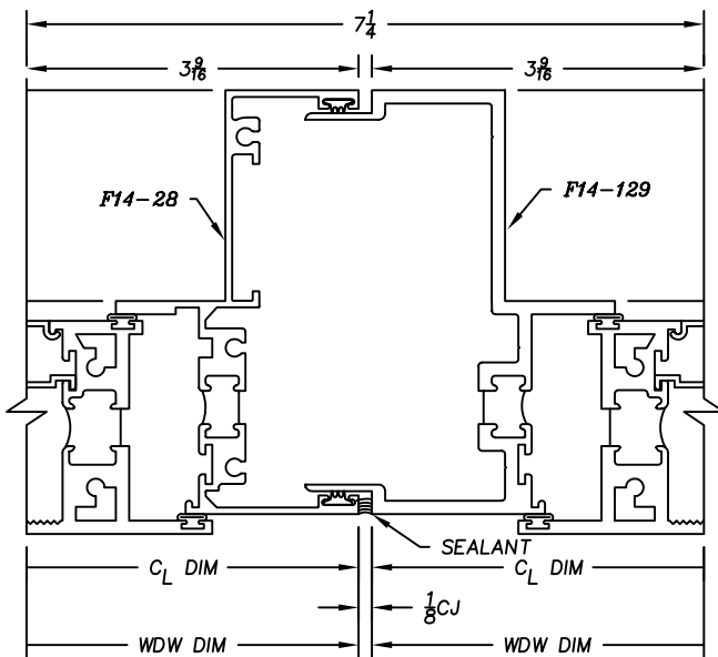
1450L SERIES - VERTICAL STACK F14-28 / F14-129
