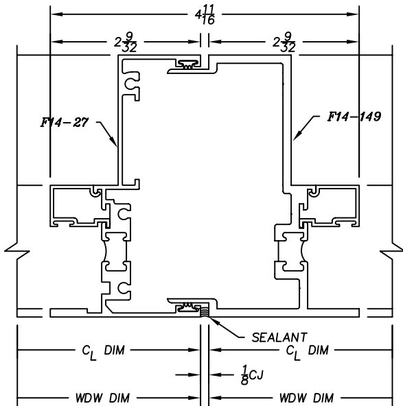
1450L SERIES - VERTICAL STACK F14-27 / F14-149
