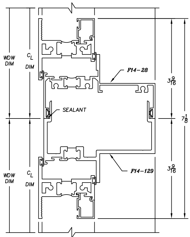
1450L SERIES - HORIZONTAL STACK F14-28 / F14-129
