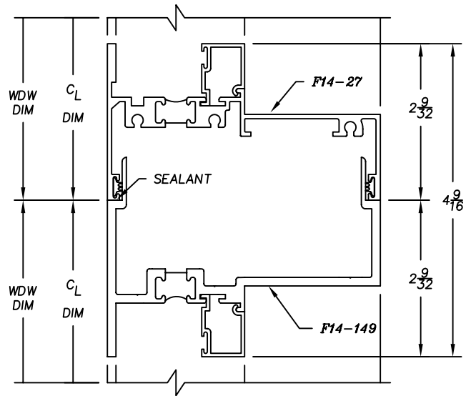
1450L SERIES - HORIZONTAL STACK F14-27 / F14-149
